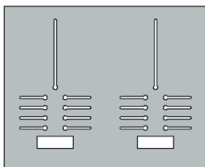
CV062602 Outflex modul målerplate 25x80cm 1 måler trafomåling 1 DIN skinne inkl avdekking
