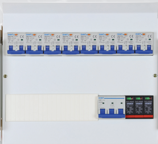
RENOVERINGSRAMME 2 RADER FOR C, D OG E-SKAP CV008204
