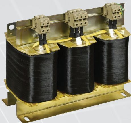
AT3 20kVA
