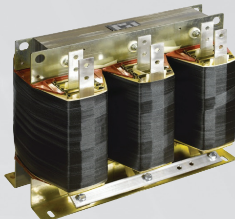
AT3 100kVA
