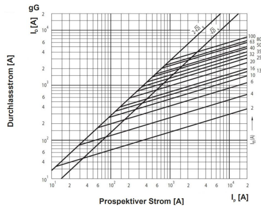
Durchlass-Kennlinie
