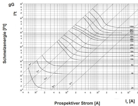
Schmelzenergie-Kennlinie
