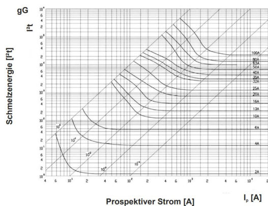
Schmelzenergie-Kennlinie
