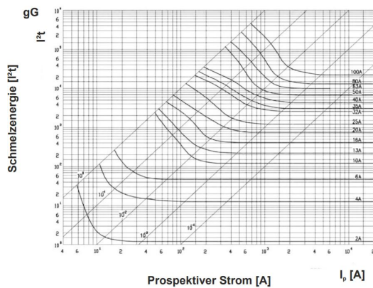
Schmelzenergie-Kennlinie
