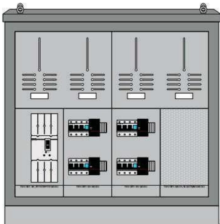
Forslag til løsning 4 målerfelt +svakstrøm
