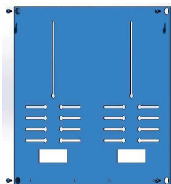
Outflex modul 50x40cm Målerplate 2 målere CV058841
