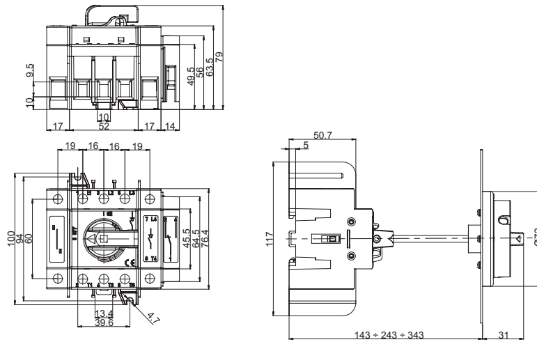
SD2 3 - 4 poli / poles
