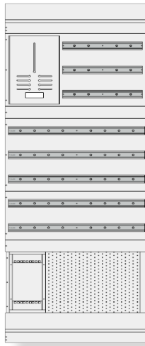
■ INNREDNING 750MM ■ VARENUMMER 990269
