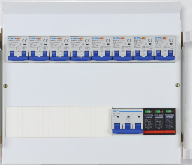
RENOVERINGSRAMME 2 RADER FOR C, D OG E-SKAP CV008204
