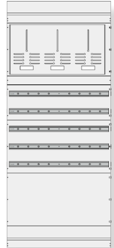
■ INNREDNING 750MM ■ VARENUMMER 990268
